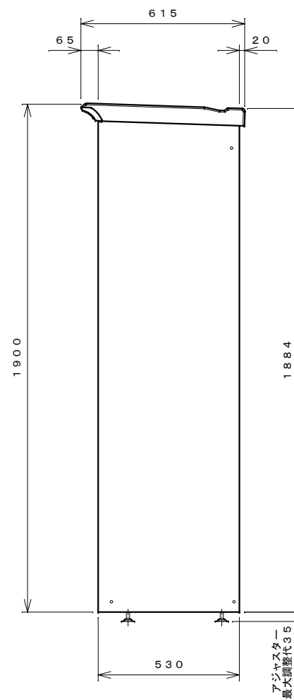
右側面図
