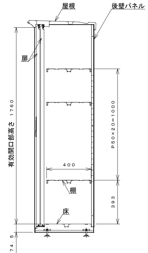
側面断面図
