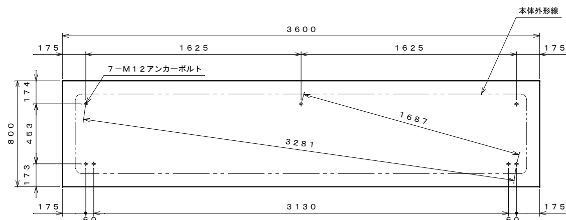
基礎伏せ図 S=1:20
