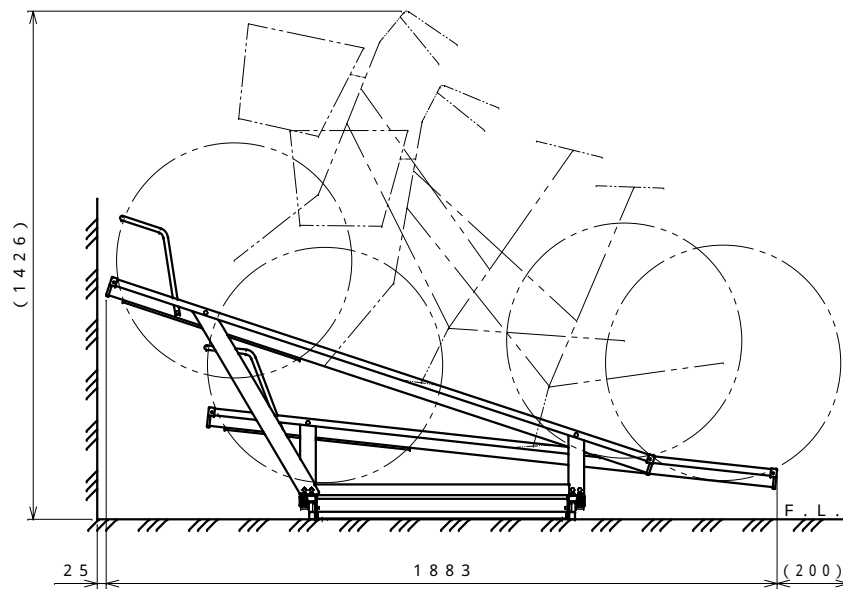
側面図 S = 1 : 15
