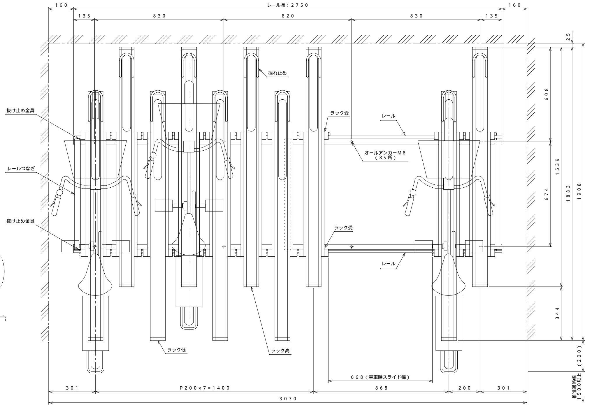
平面図 S = 1 : 10
