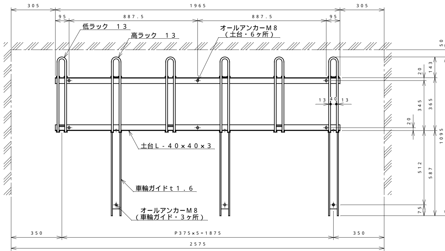
平面図 S = 1 : 15
