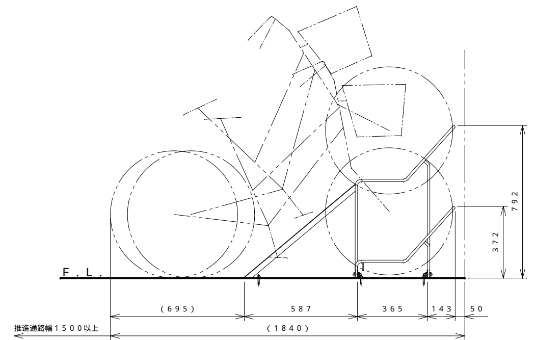
側面図 S = 1 : 20
