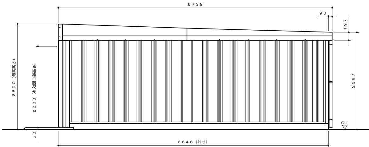
側面図 S=1:40
