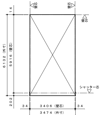
面積求積図 S = 100
