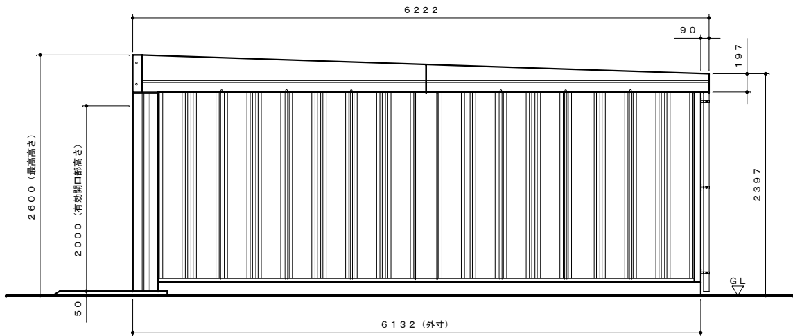
側面図 S = 1 : 40
