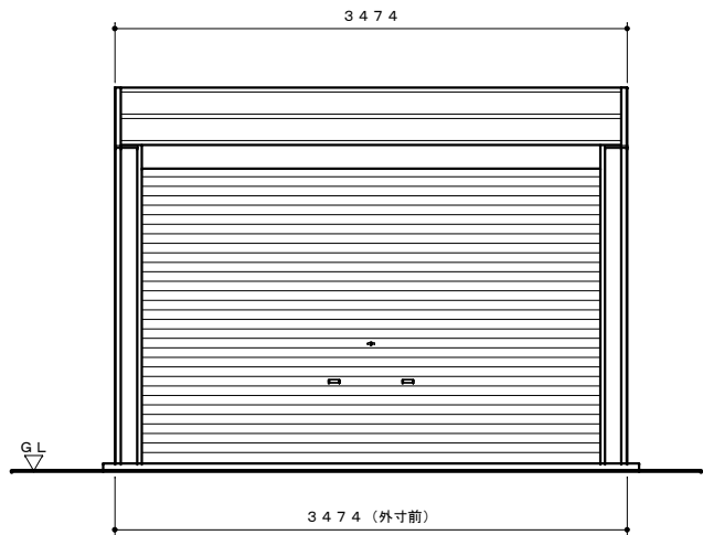
正面図 S = 1 : 40
