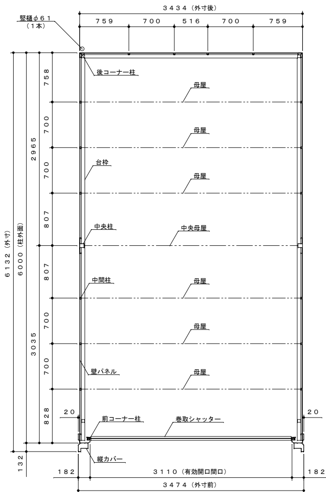
平面図 S = 1 : 40
