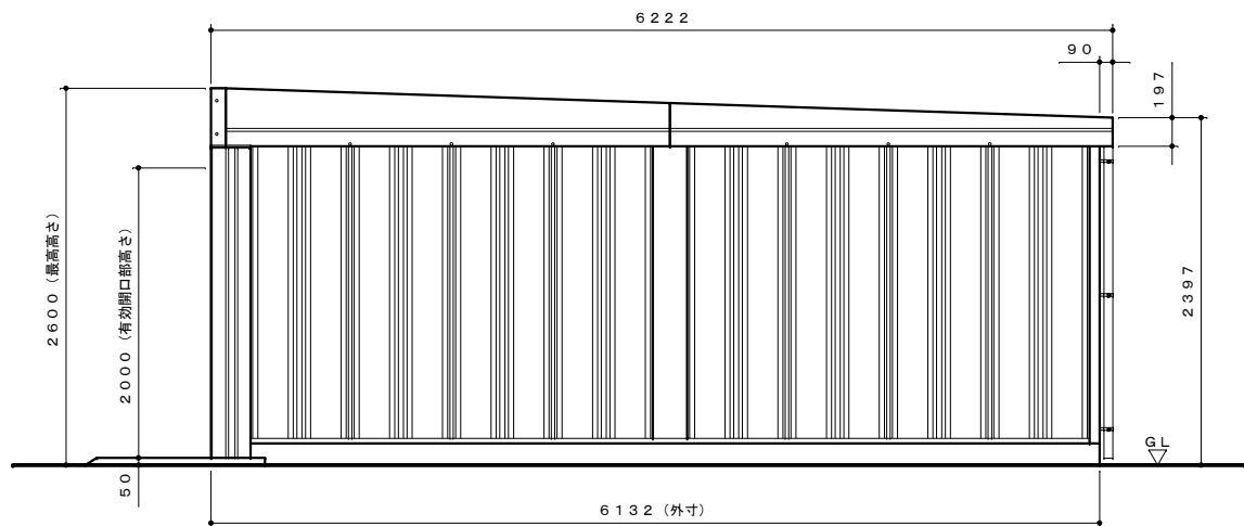
側面図 S = 1 : 4 0
