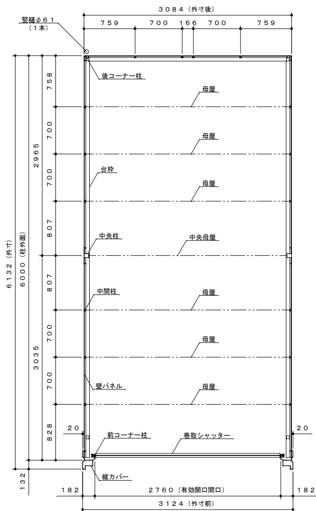
平面図 S = 1 : 4 0
