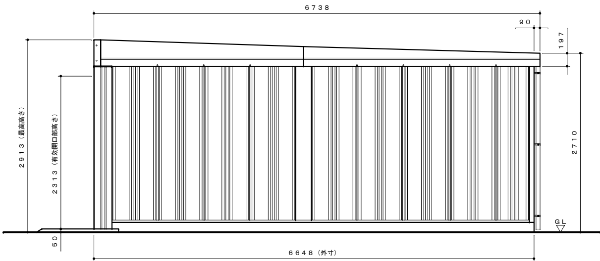
側面図 S=1:40
