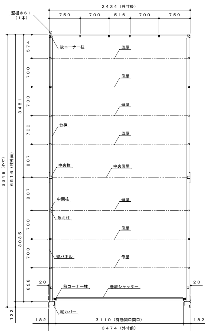
平面図 S=1:40
