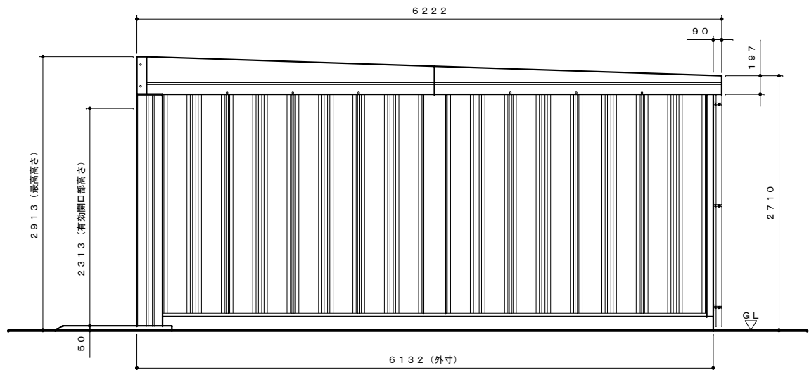
側面図 S = 1 : 40
