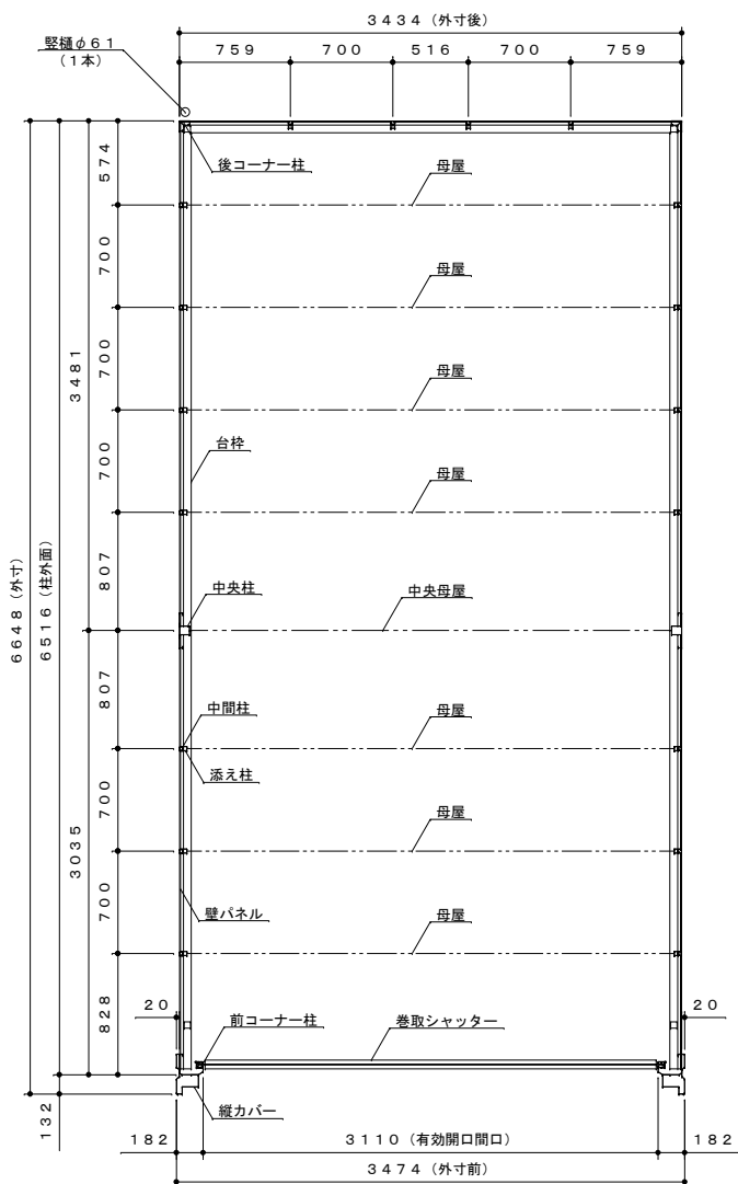
平面図 S = 1 : 40
