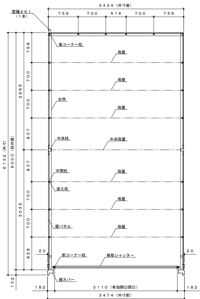
平面図 S=1:40
