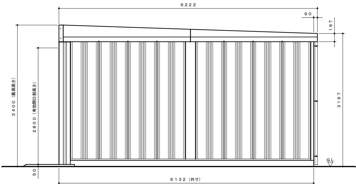
側面図 S=1:40
