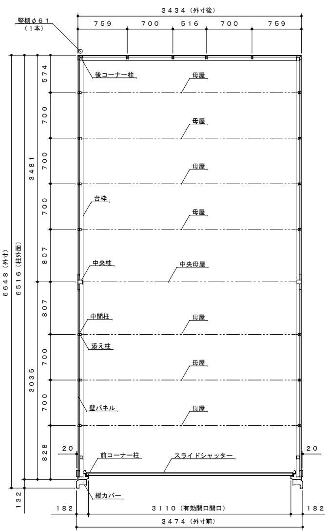
平面図 S=1:40
