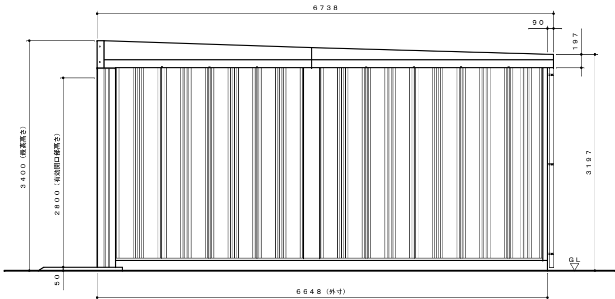
側面図 S=1:40
