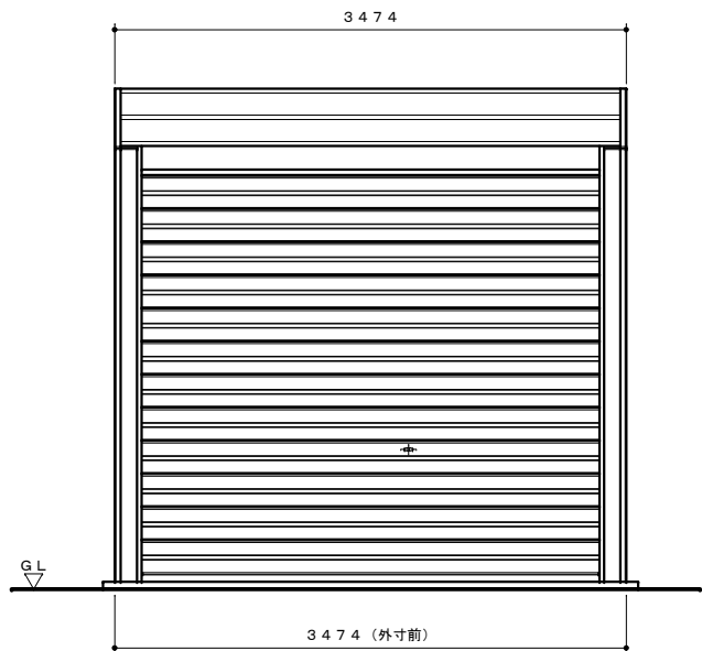
正面図 S=1:40
