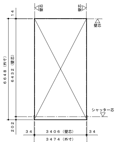
面積求積図 S=100
