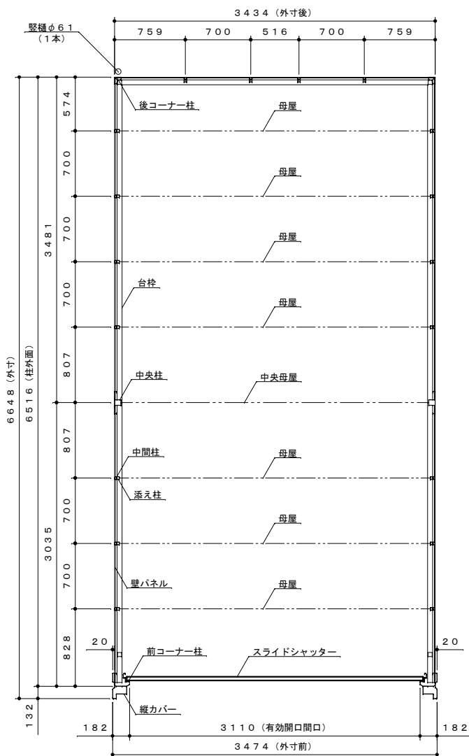
平面図 S=1:40
