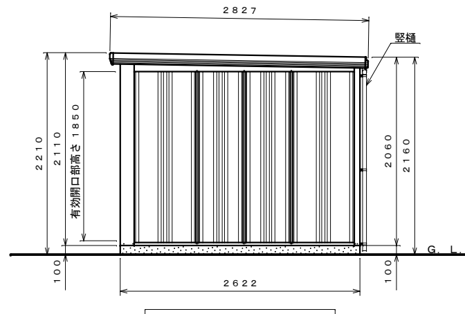
側面図 S=1:40
