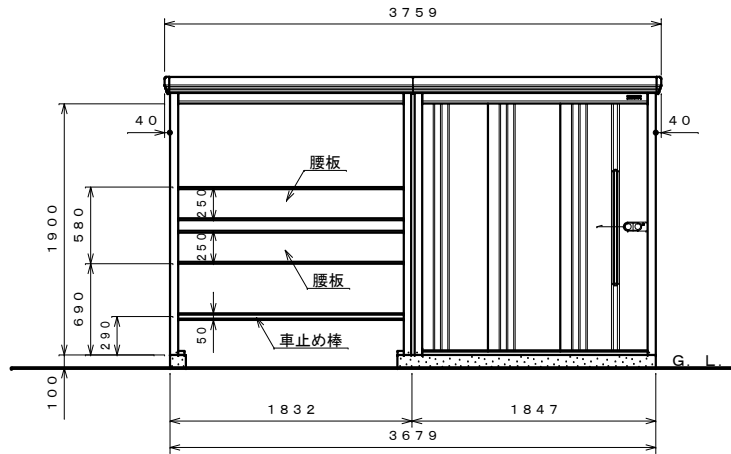
正面図 S=1:40
