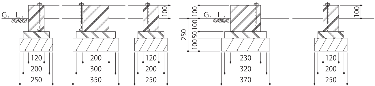
正面断面図
