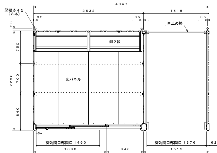
平面図 S=1:30
