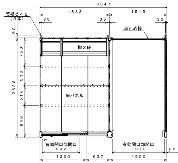
平面図 S=1:40
