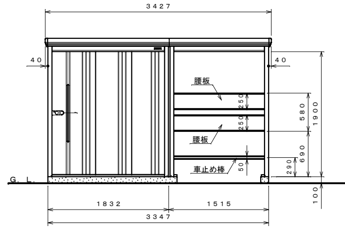
正面図 S=1:40
