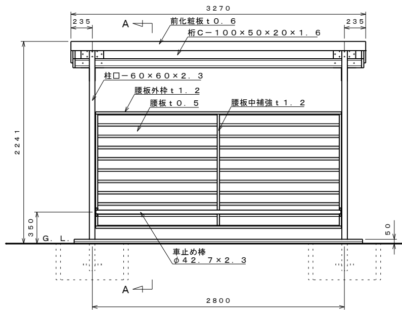
正面図 S=1:30
