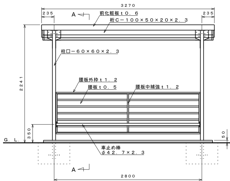
正面図 S=1:30
