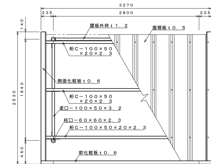
平面図 S=1:30
