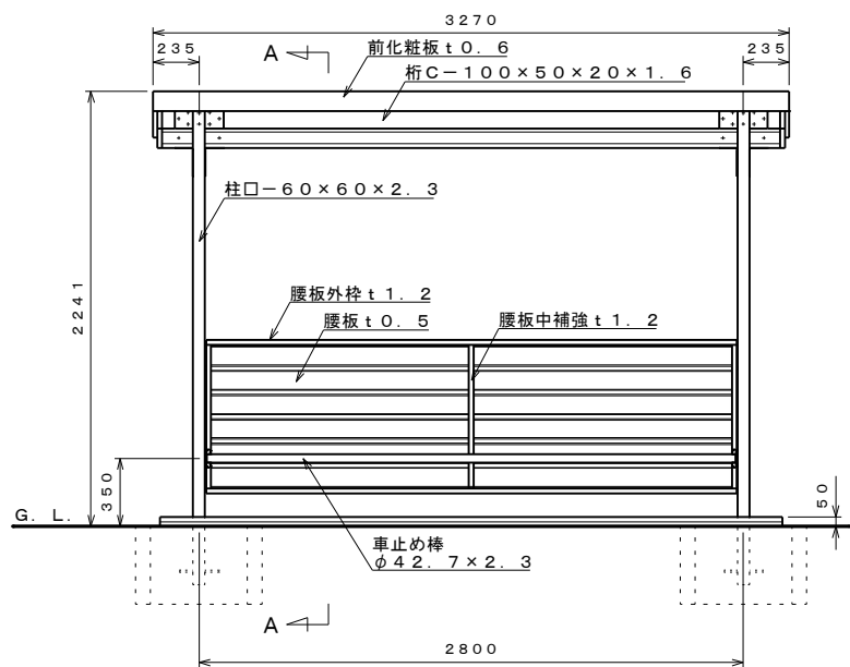
正面図 S=1:30
