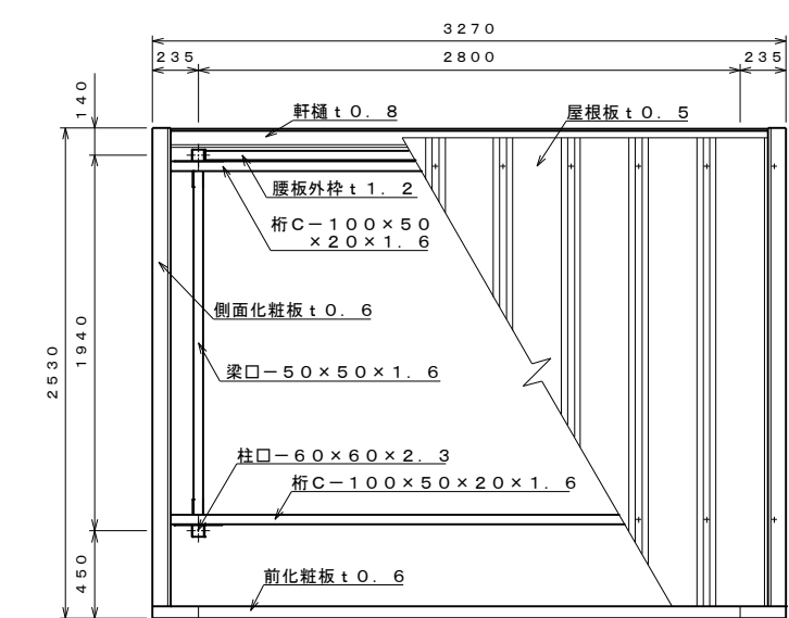
平面図 S=1:30
