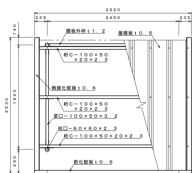
平面図 S=1:30
