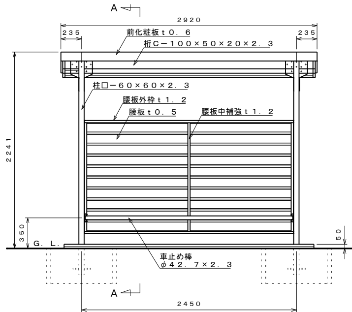
正面図 S=1:30
