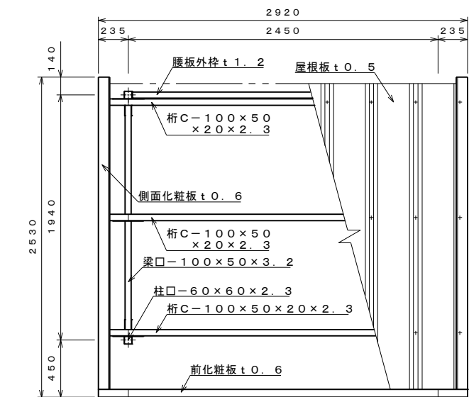
平面図 S=1:30
