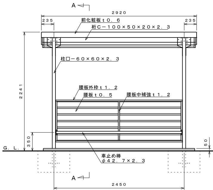
正面図 S=1:30
