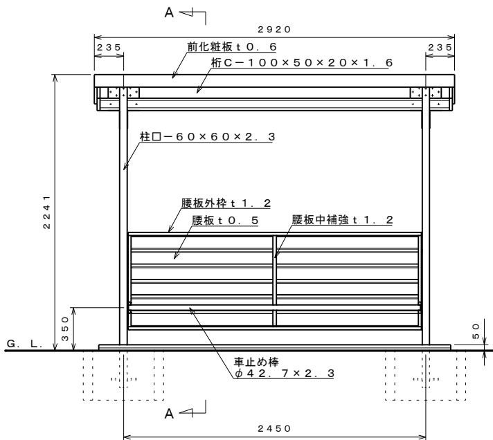
正面図 S=1:30
