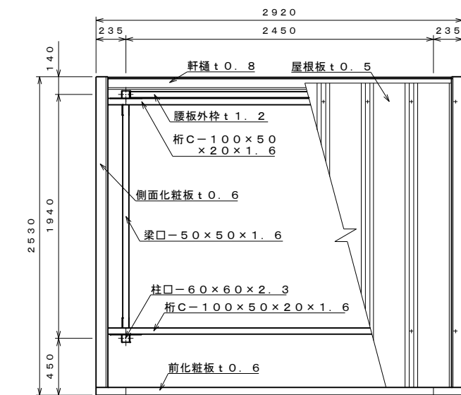
平面図 S=1:30
