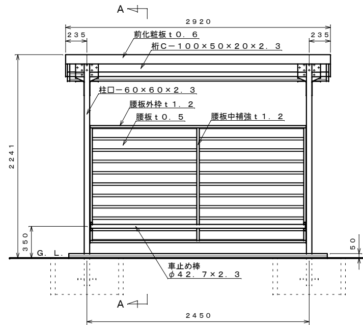
正面図 S=1:30
