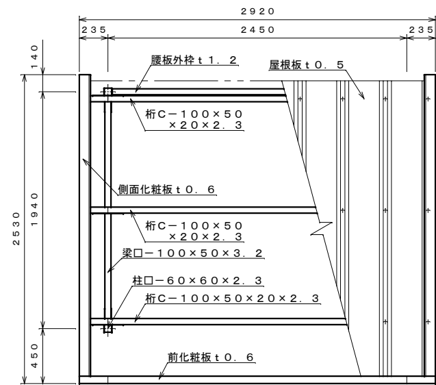
平面図 S=1:30
