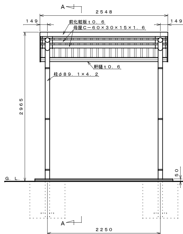
正面図 S=1:30
