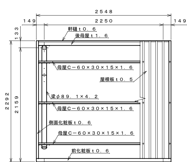
平面図 S=1:30
