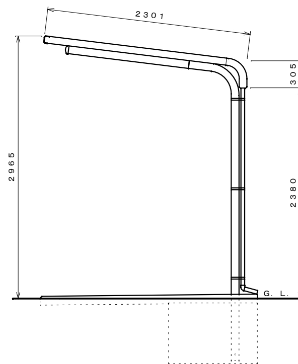
側面図 S=1:30
