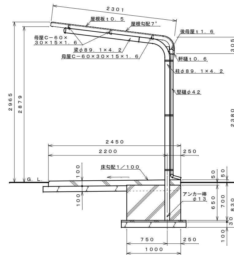
A-A断面図 S=1:30 コンクリート強度: F_c 21 \text{ N/mm}^2 以上
