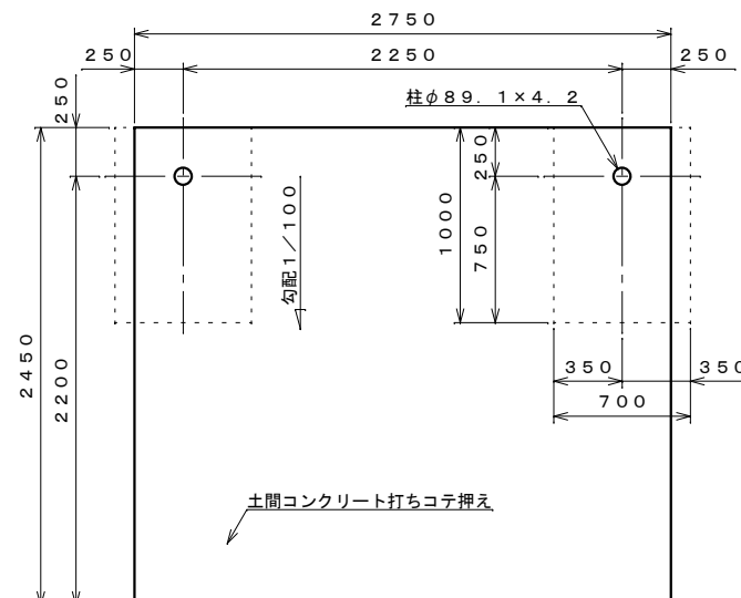
基礎伏せ図 S=1:30 (注: この基礎は標準を示しています。現場の実情に合わせて、ご設計下さい。)
