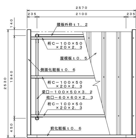
平面図 S=1:30
