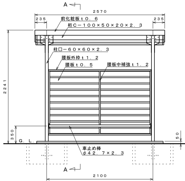
正面図 S=1:30
