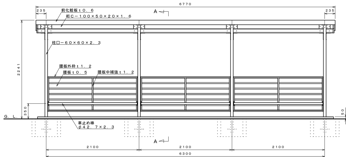
正面図 S=1:30
