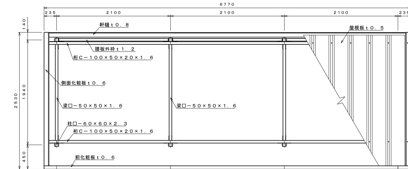
平面図 S=1:30
