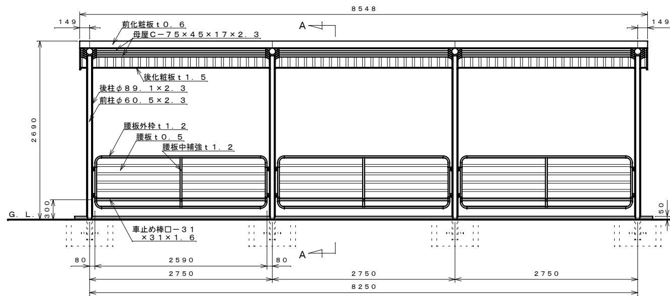
正面図 S=1:40
