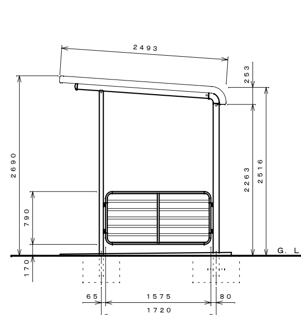
側面図 S=1:40
