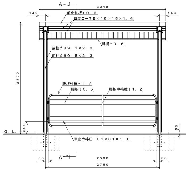
正面図 S=1:30
