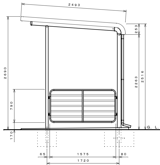
側面図 S=1:30
