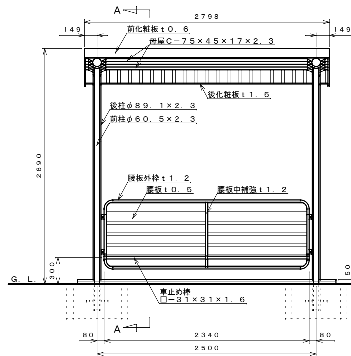
正面図 S=1:30
