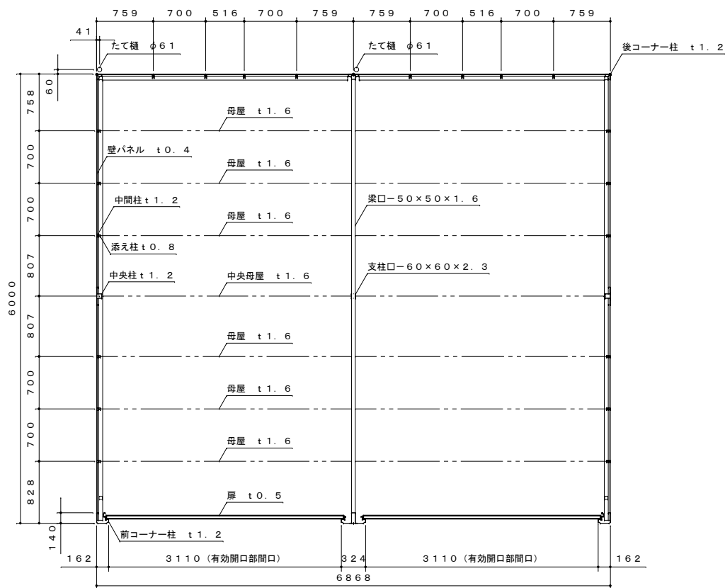
平面図 S=1:50
