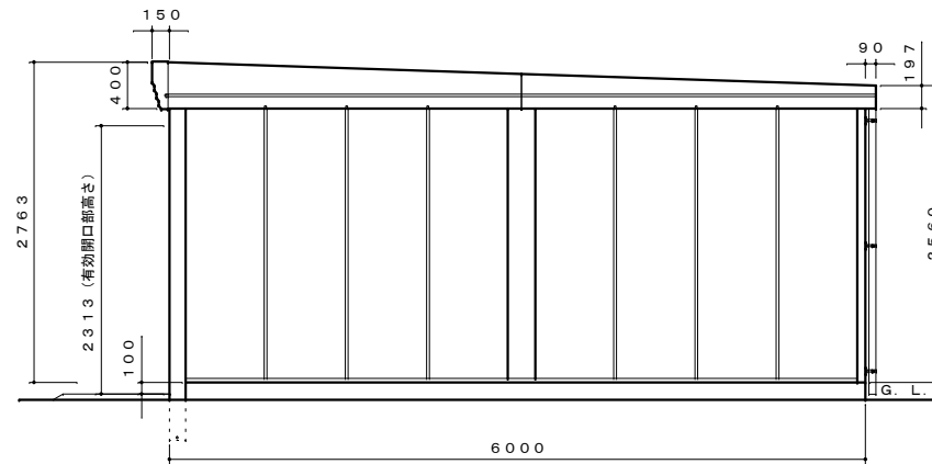
側面図 S=1:50
