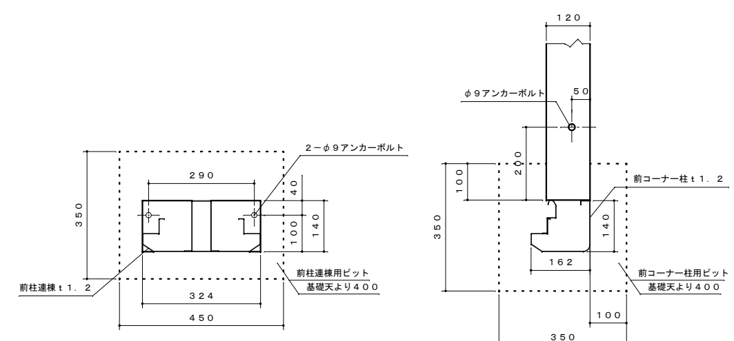
柱脚伏図 S=1:10
