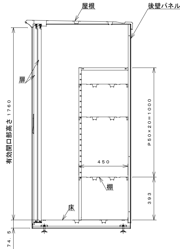
側面断面図
