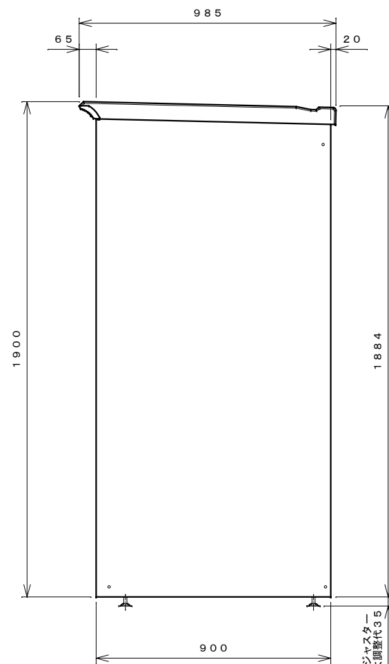
右側面図
