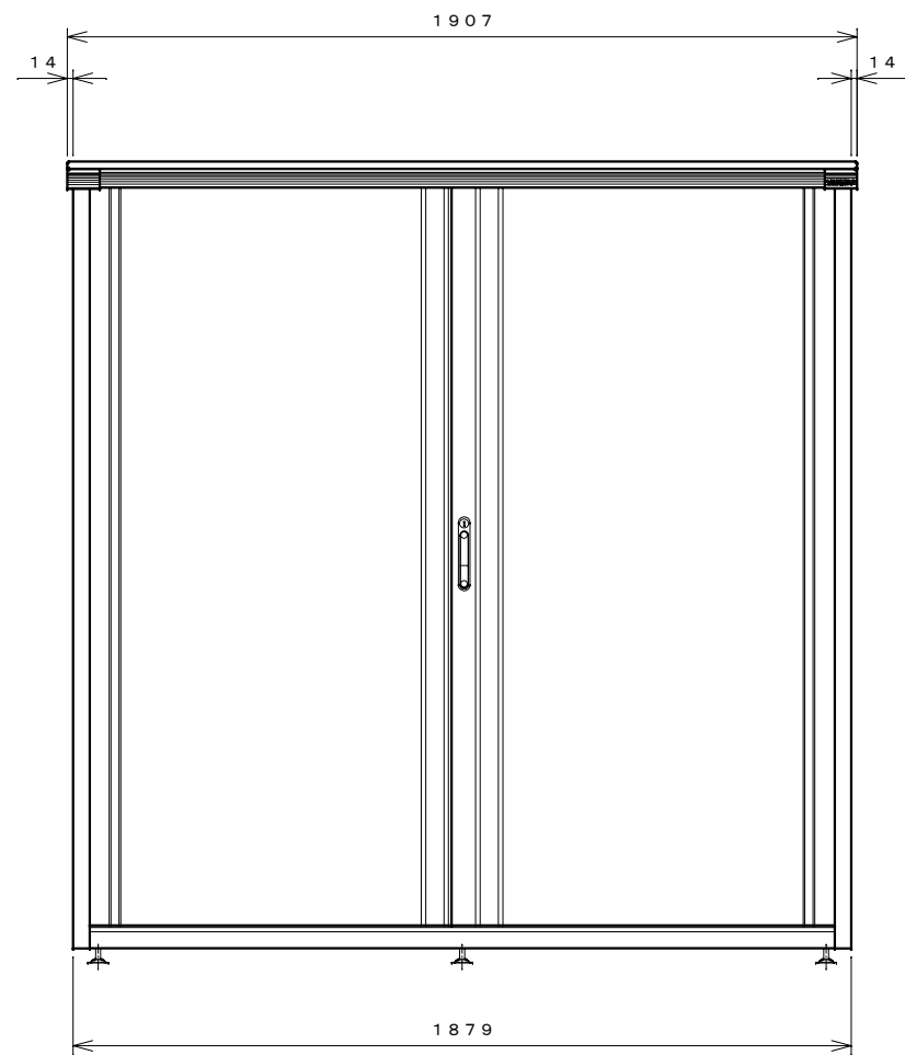
正面図
