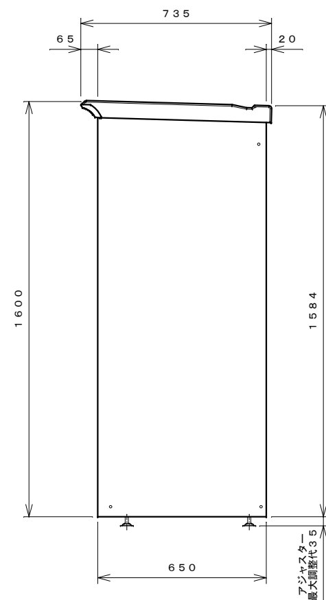
右側面図
