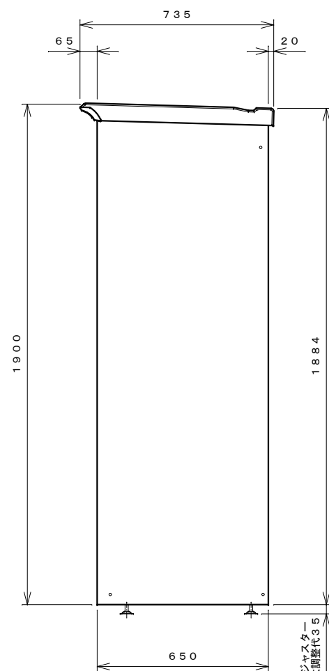
右側面図
