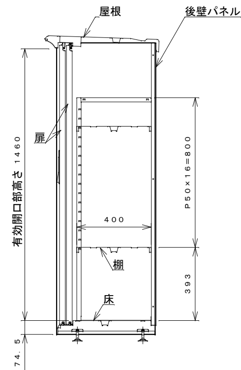
側面断面図
