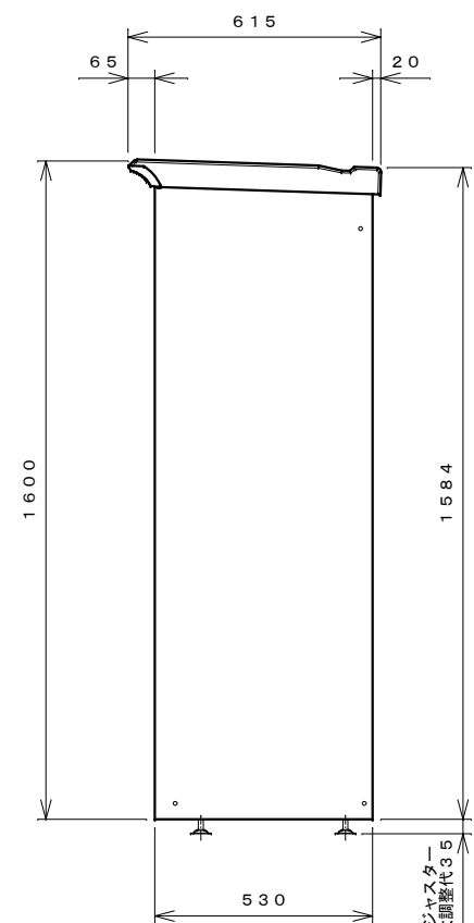
右側面図
