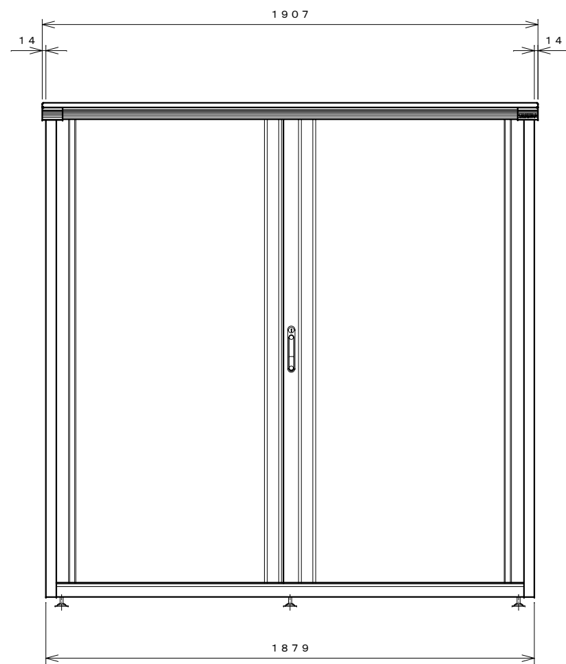
正面図
