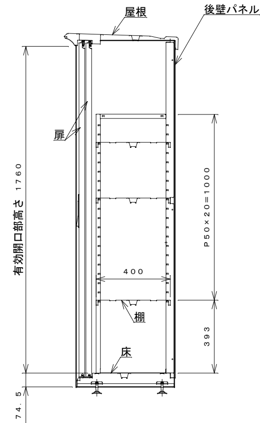
側面断面図
