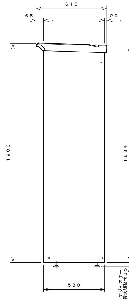
右側面図
