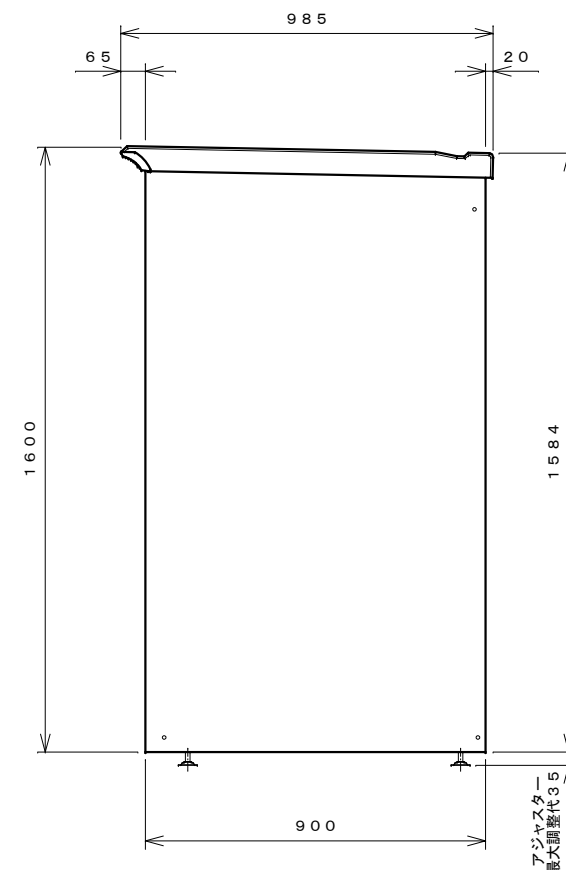
右側面図
