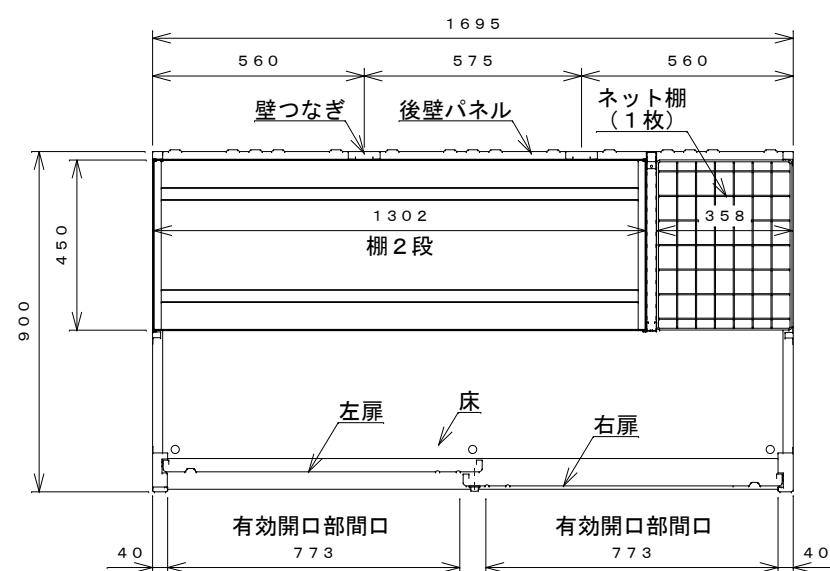
平面断面图
