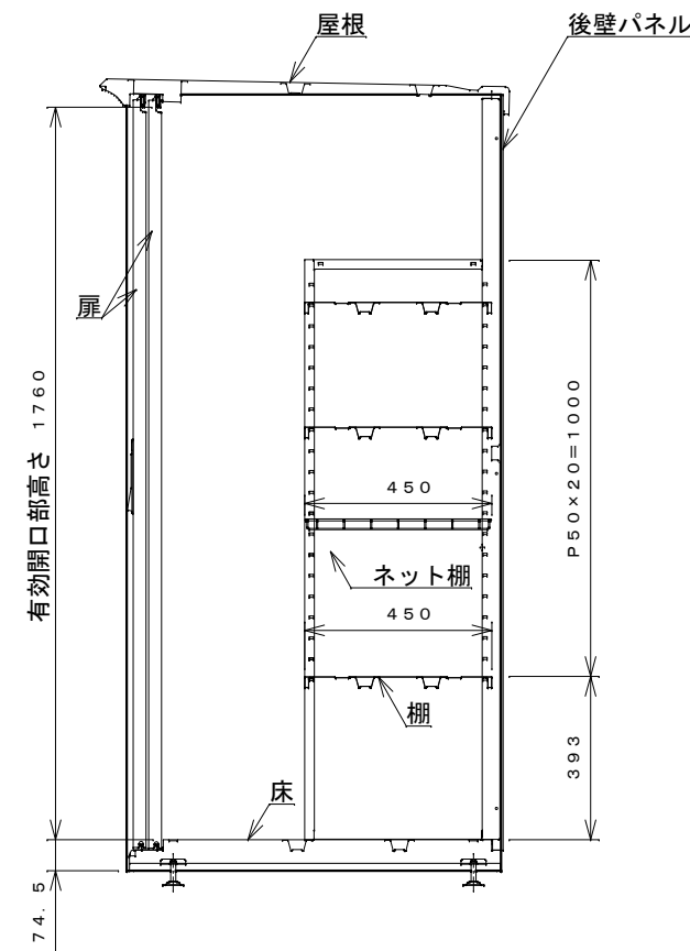
側面断面図
