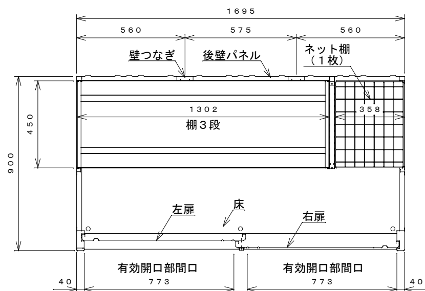
平面断面図
