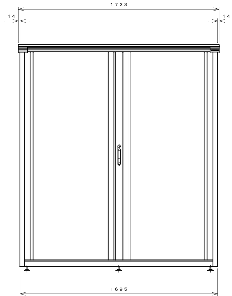
正面図
