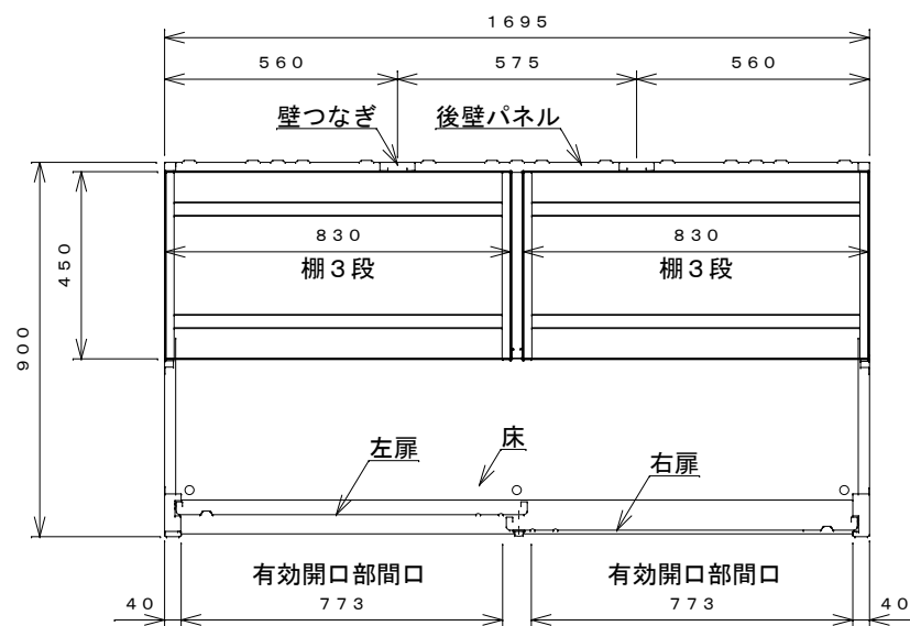
平面断面図
