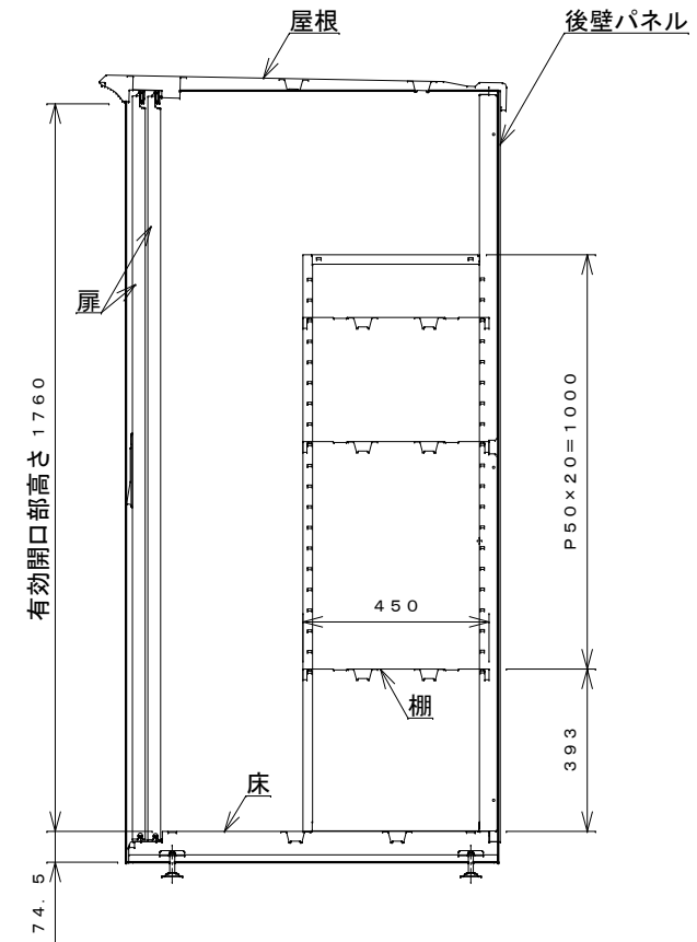
側面断面図
