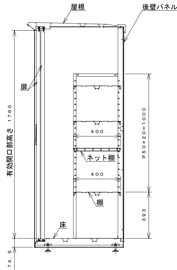
側面断面図
