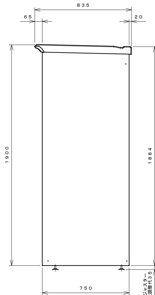
右側面図
