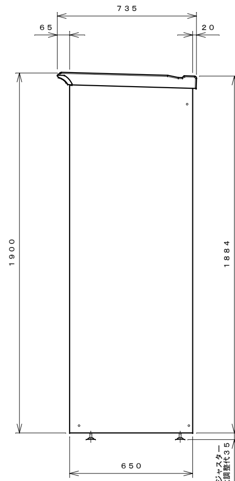
右側面図
