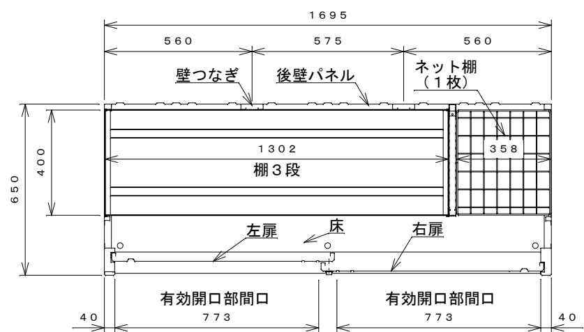
平面断面図
