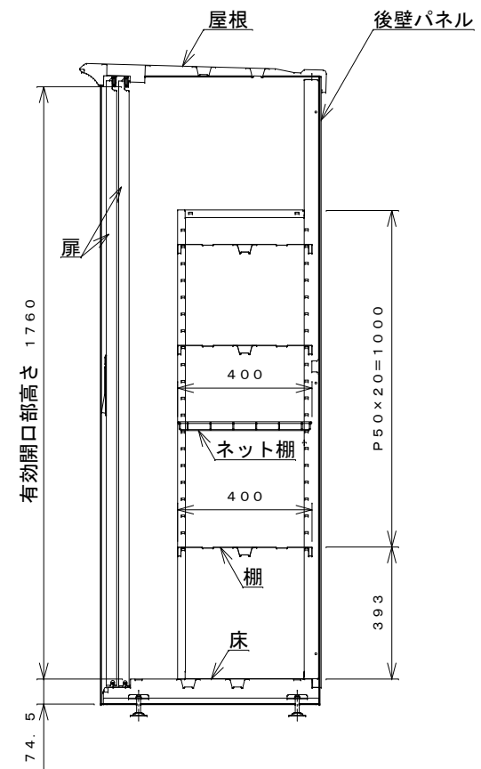
側面断面図
