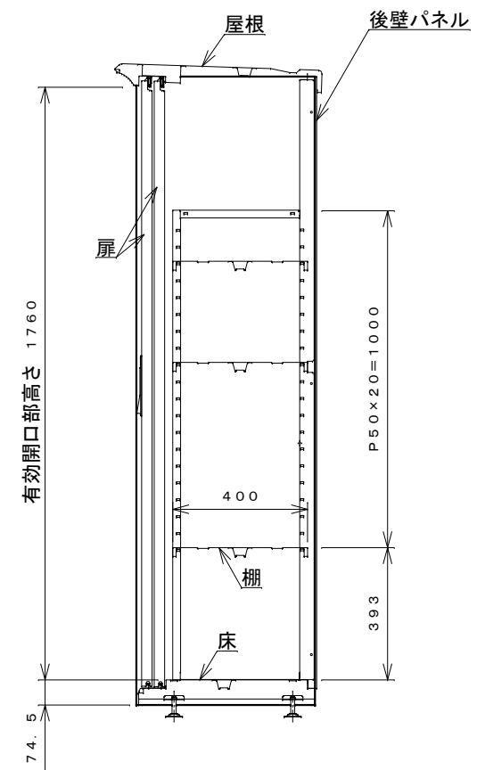
側面断面図
