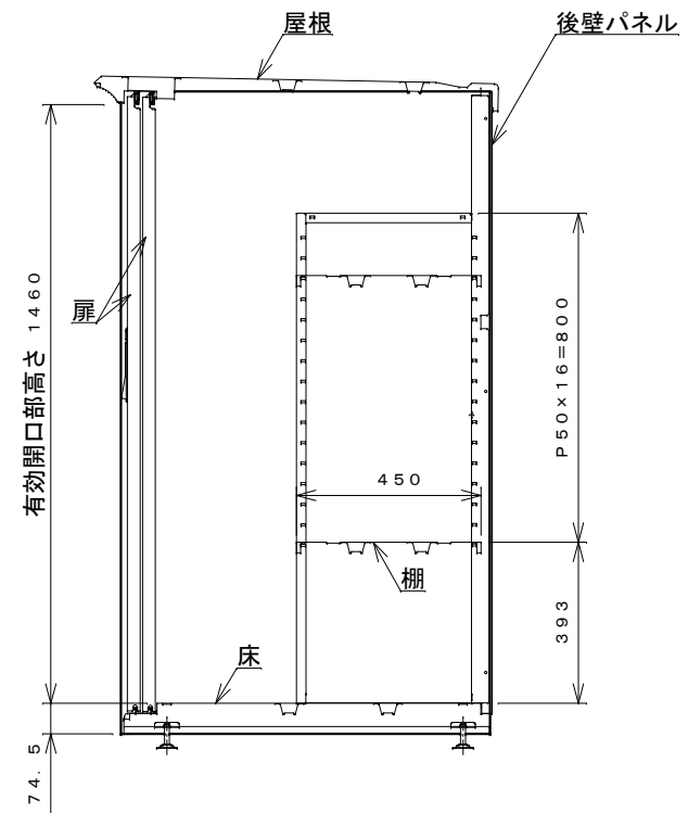
側面断面図
