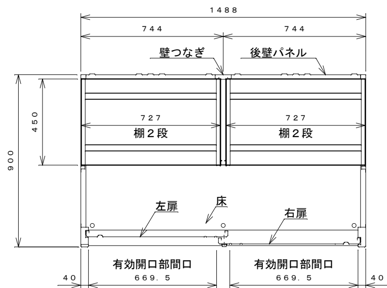
平面断面図
