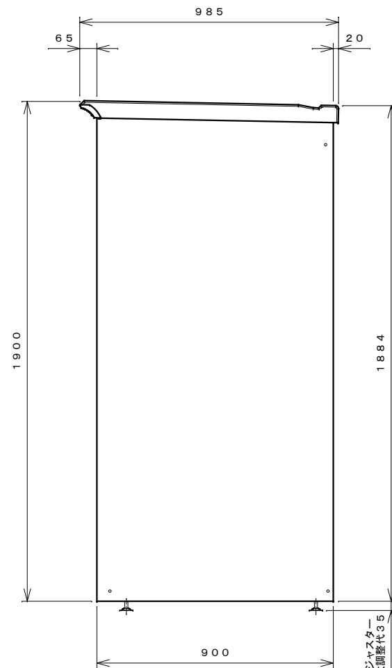
右側面図
