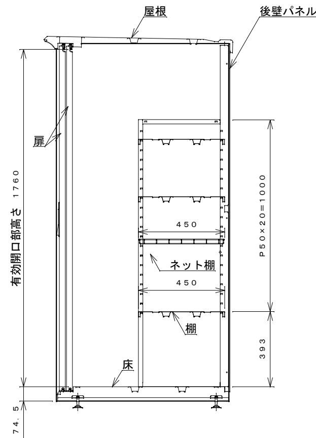
側面断面図
