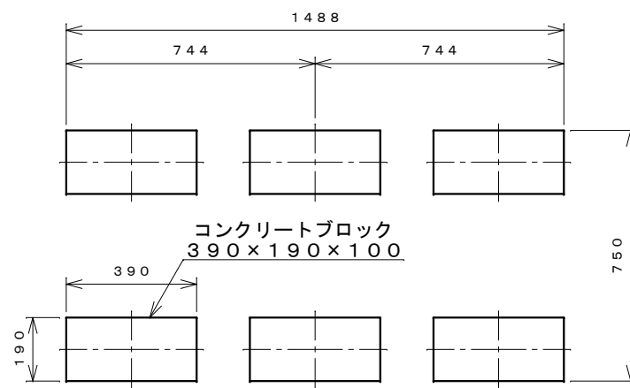
ブロック並べ図
