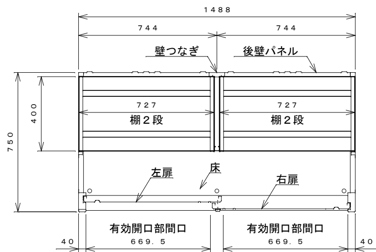
平面断面図
