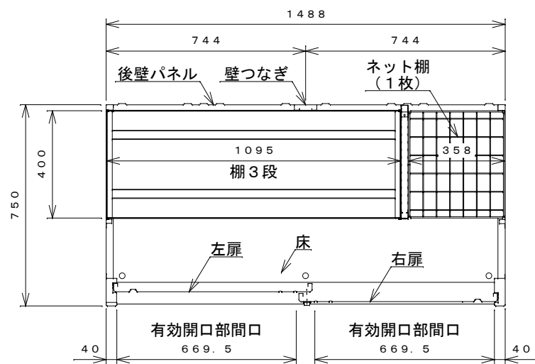
平面断面図
