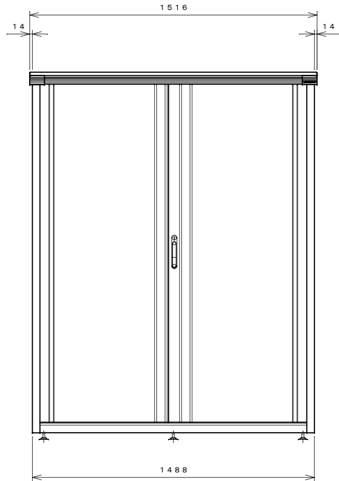
正面図
