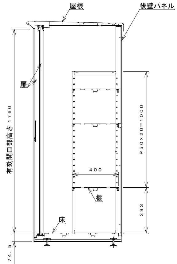
側面断面図
