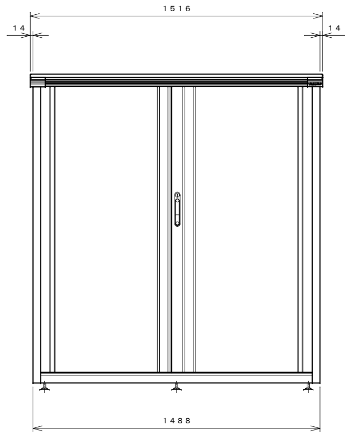
正面図
