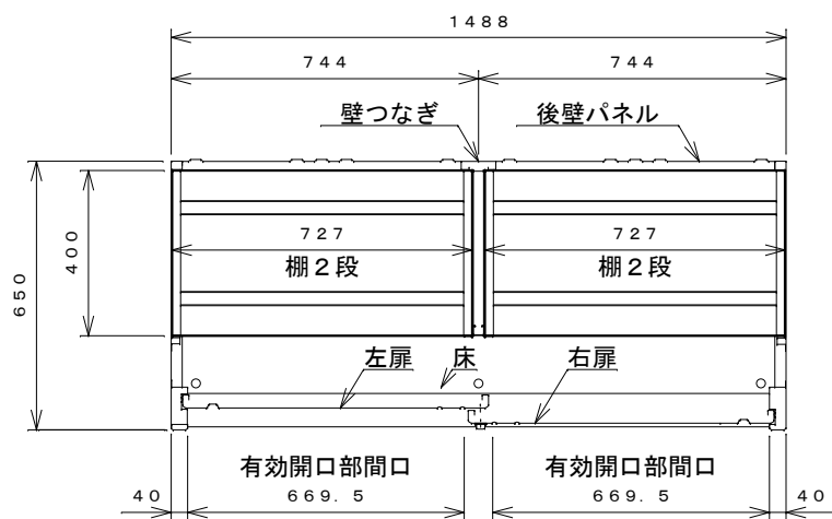
平面断面図
