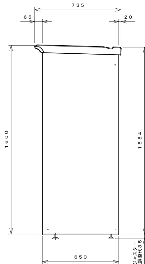
右側面図
